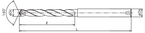
X形シンニング X thinning (Dc < 4)
